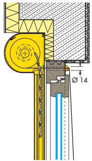
Der VOKA mit Rundkasten in der Sturznische eingebaut.
