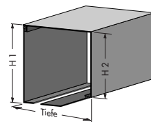
Standardkasten, rollverformt oder stranggepresst
