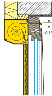
Die Situation beim nachträglichen Einbau mit Sichtblende (Gurtaustritt oben ist Option).
