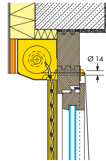
Einbaudetail mit Stockaufdoppelung und Putzblende. Dadurch ragt der Rollladenkasten nicht mehr ins Fenster.
