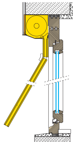
Ausstellscharnier
