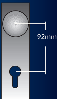
Haustür
