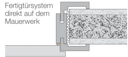
Fertigtürsystem über Stahlzarge
